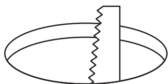
otwór pod oprawę ø120-130mm
